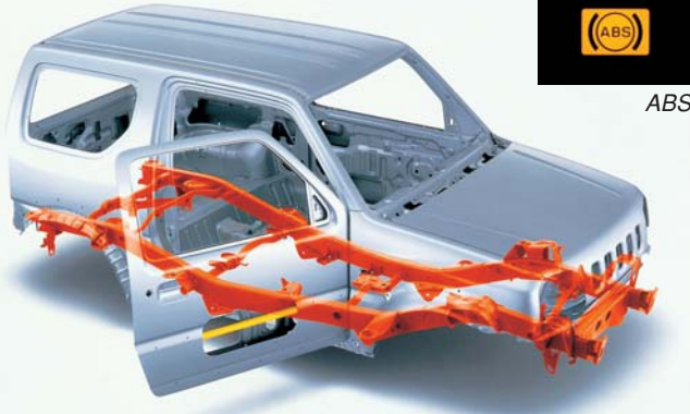
Masszív alvázszerkezet – három részből álló, létraszerű alváz
