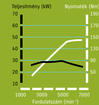
Az 1 literes motor teljesítménygörbéje (67 LE/50 kW)
