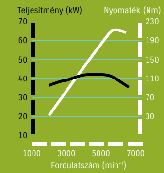
Az 1,2 literes motor teljesítménygörbéje (93 LE/69 kW)
